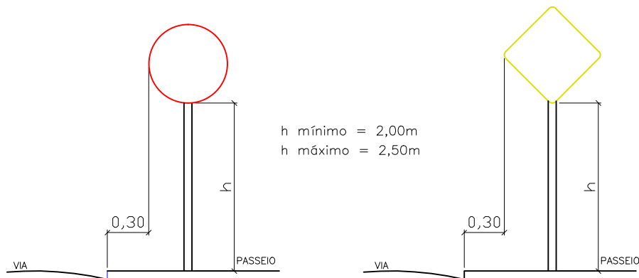
DETALHES PARA LOCAÇÃO DE PLACAS
