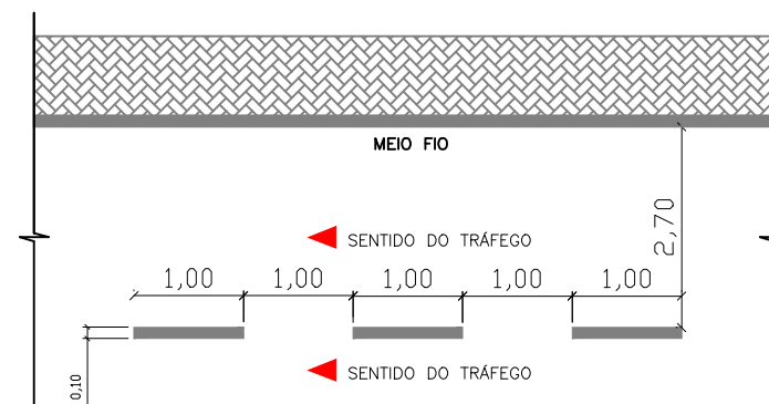
DETALHE DE LINHA DE FECHAMENTO PARA ESTACIONAMENTO SIMPLES PARALELO AO MEIO FIO COM DEMARCAÇÃO AO LONGO DO TRECHO.
