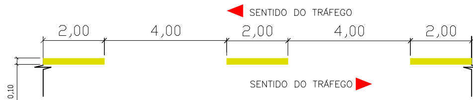
DETALHE DE LINHA SIMPLES SECCIONADA DE DIVISÃO DE FLUXOS OPOSTOS FLUXOS DE SENTIDO ÚNICO: COR BRANCA
