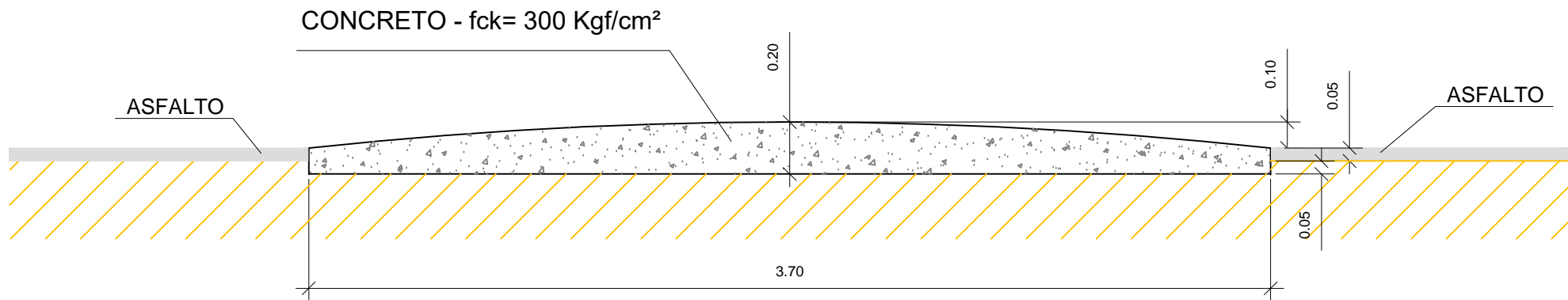
CORTE TRANSVERSAL
