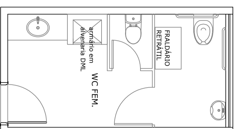
BANHEIROS BLOCO 02 PROPOSTA REFORMA
