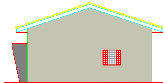
FACHADA 02 ESC. 1/150
