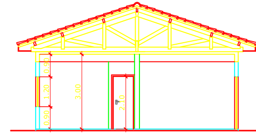
CORTE BB ESC. 1/150
