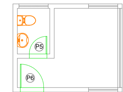
GUARITA - CONSTRUÇÃO ESCALA: 1/75
