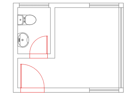
GUARITA - DEMOLIÇÃO ESCALA: 1/75
