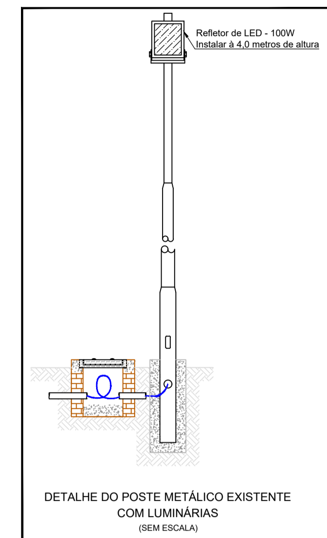
ESCALA SEM ESCALA DETALHE DA INSTALAÇÃO DO POSTE E REFLETORES DE LED
