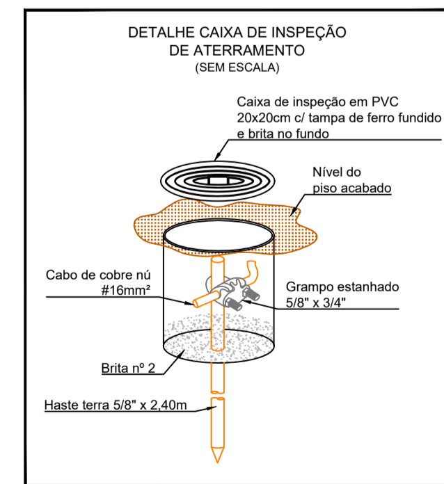
ESCALA SEM ESCALA DETALHE DA CAIXA DE INSPEÇÃO DO ATERRAMENTO
