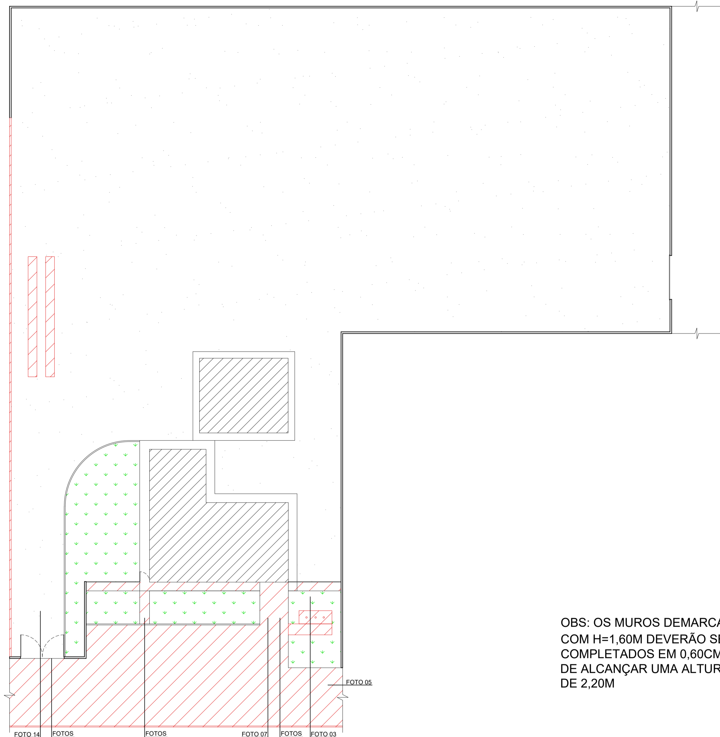
IMPLANTAÇÃO - DEMOLIÇÃO ESCALA: 1/200
