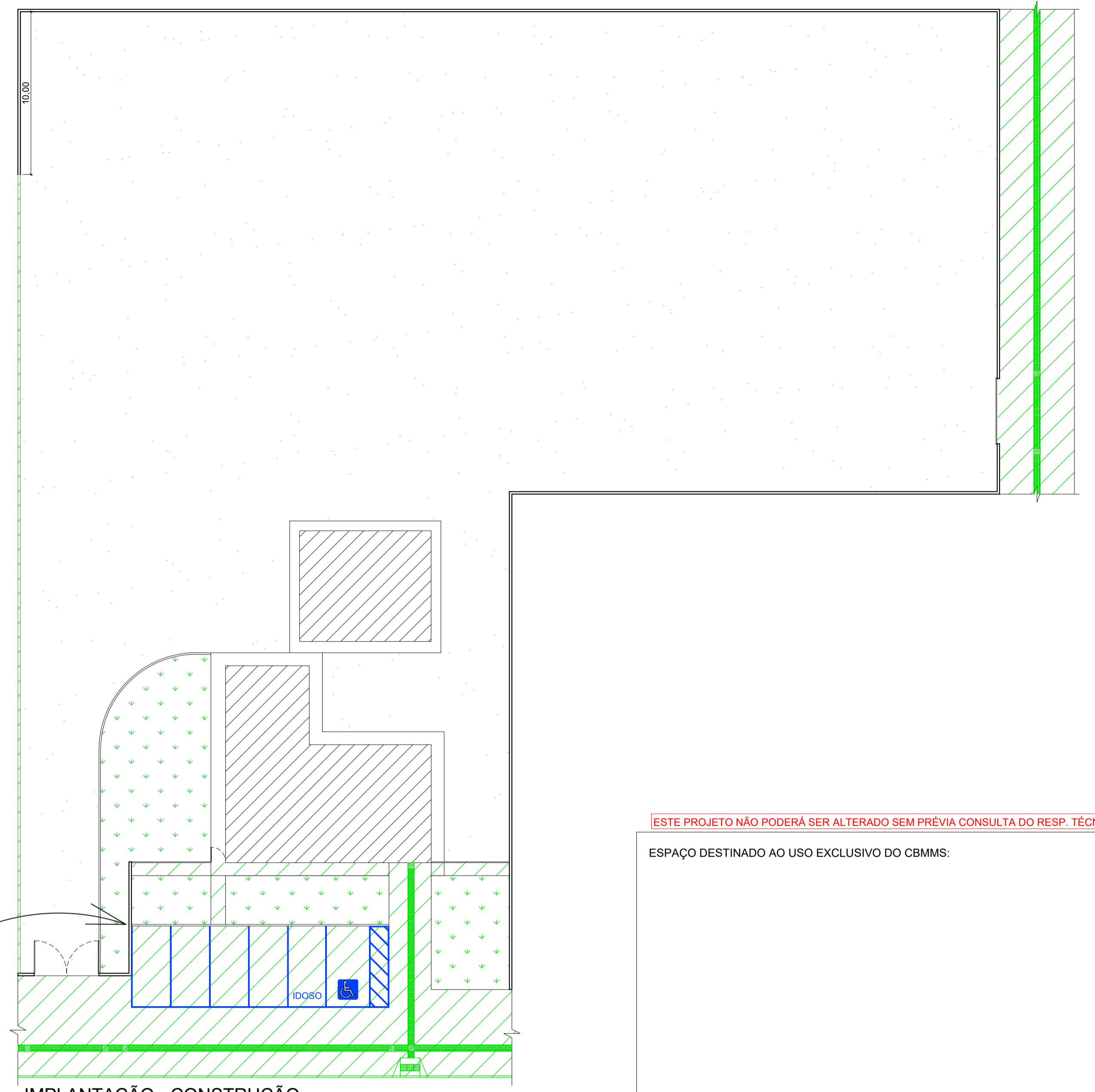
IMPLANTAÇÃO - CONSTRUÇÃO ESCALA: 1/200
