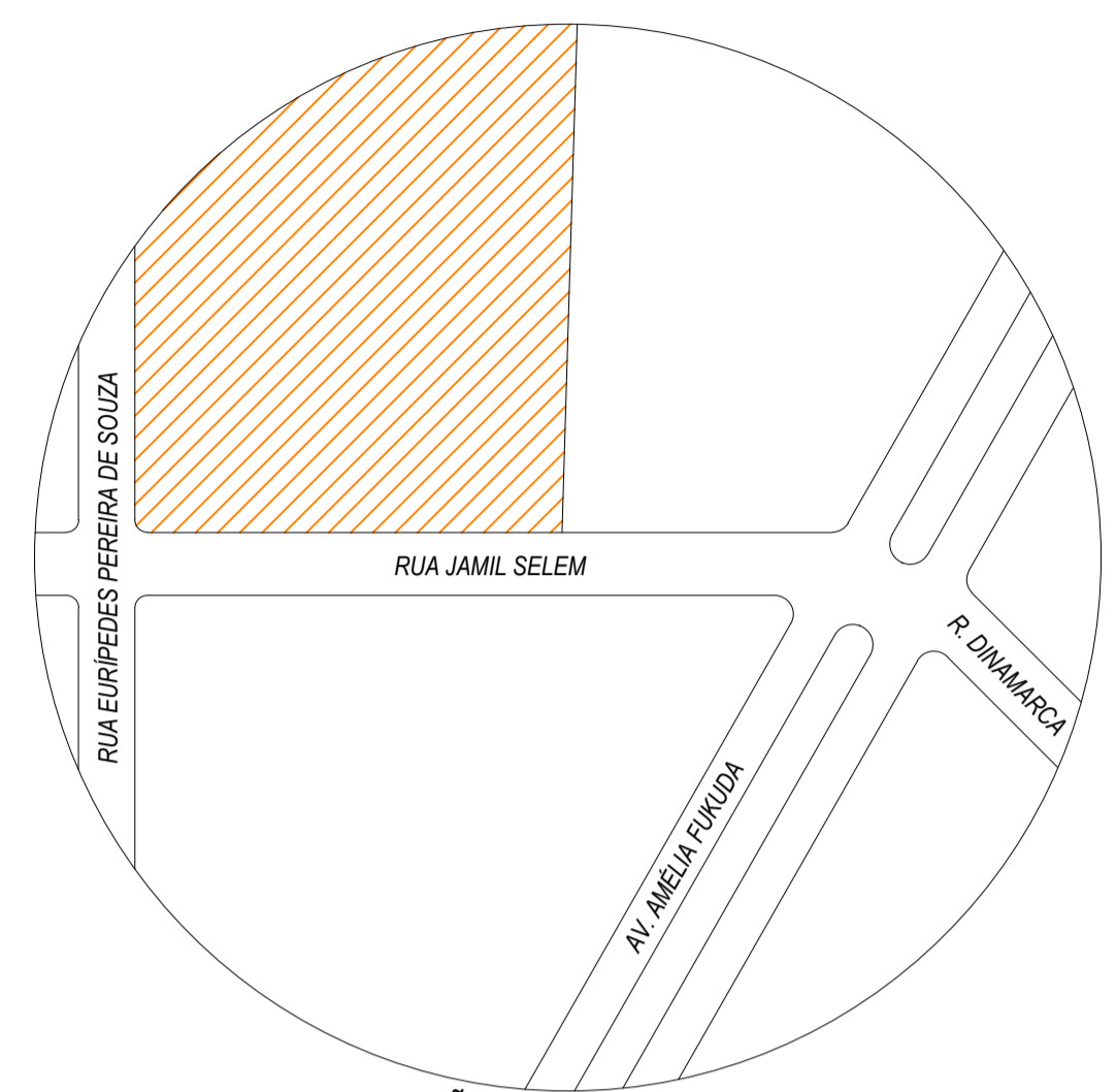
PLANTA DE SITUAÇÃO ESCALA: 1/1250 LEGENDA TERRENO DA AGÊNCIA
