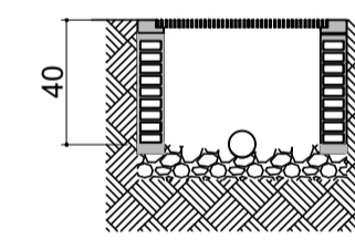
CAIXA DE ÁGUA PLUVIAL Esc 1:50
