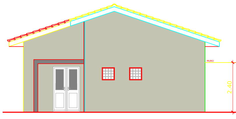
FACHADA 02 ESC. 1/100
