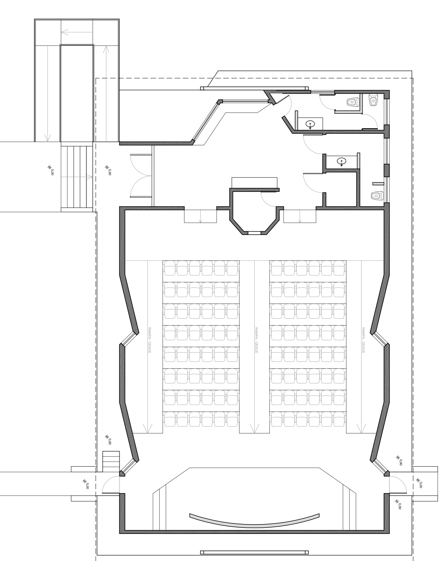
PLANTA BAIXA ATUAL - AUDITÓRIO DETRAN/MS Escala: 1/100
