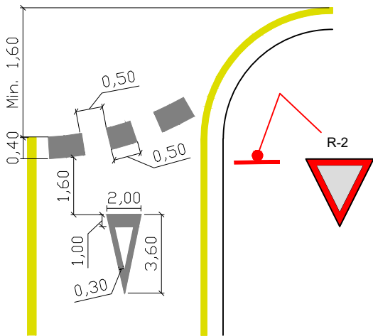
LINHA DE PREFERÊNCIA E SÍMBOLO INDICATIVO COM VIA QUE TEM PREFERÊNCIA, VEL. < 60KM/H
