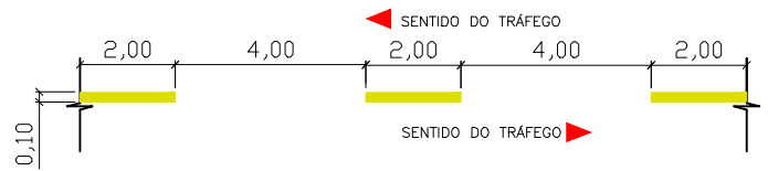
DETALHE DE LINHA SIMPLES SECCIONADA DE DIVISÃO DE FLUXOS OPOSTOS. FLUXOS DE SENTIDO ÚNICO: COR BRANCA
