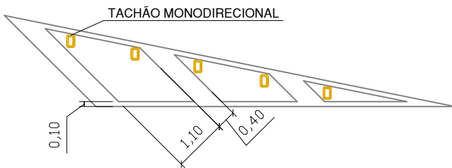
DETALHE DE ZEBRADO
